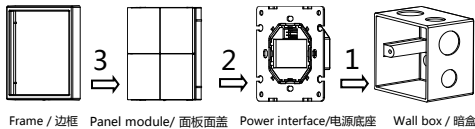
Figure 5. Installation 图 5. 安装图
